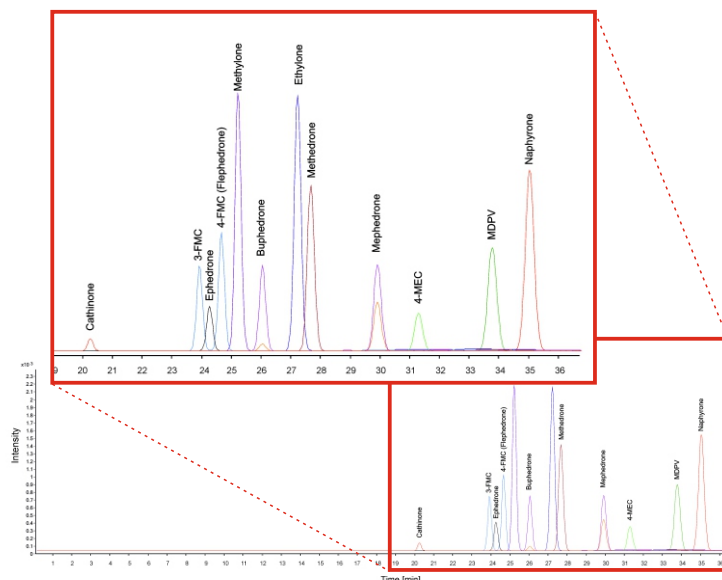
Separace zneužívaných "designer" kationů s pomocí CE-ESI-MS/MS.
